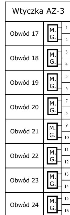
Karta wejść pomiarowych SEKCJA 1
