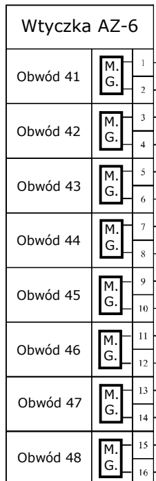
Karta wejść pomiarowych SEKCJA 2
