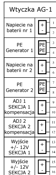
Karta generatora Bateria 1 i 2
