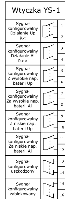
Karta wyjść sterowniczych i sygnalizacyjnych
