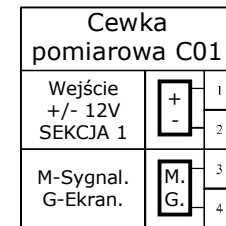
C01-C32 - SEKCJA 1 C33-C64 - SEKCJA 2
