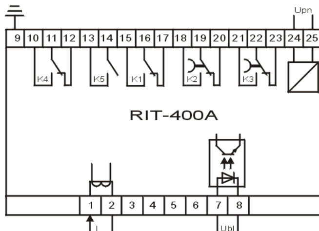
Rys. 1a. Schemat połączeń przekaźnika RIT-400A-01/05
