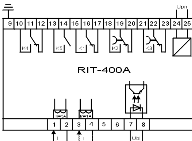
Rys. 1b. Schemat połączeń przekaźnika RIT-400A-15
