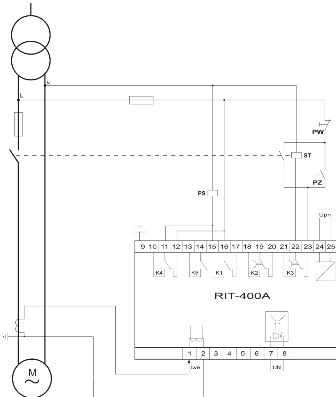
Rys. 4 Schemat połączeń zewnętrznych przełącznika RIT-400A w układzie zabezpieczenia zwarciovie silnika niskiego napięcia.
