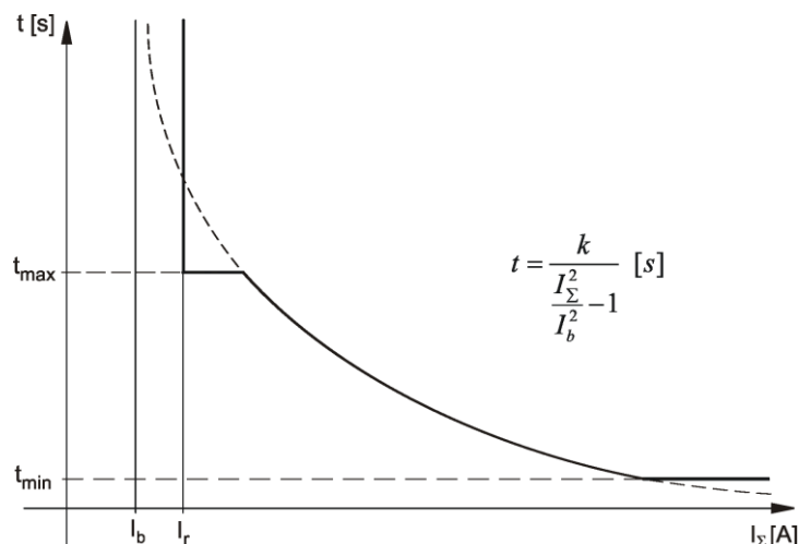
Rysunek 2. Przykładowa charakterystyka czasowa zależna zabezpieczenia I_{p2} > .
